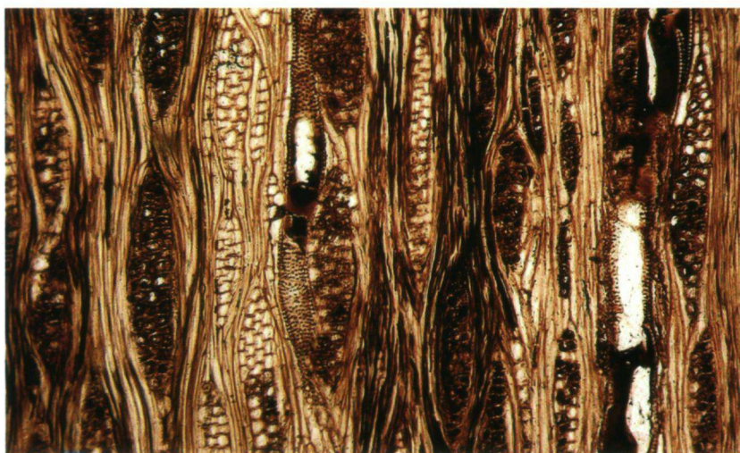
AFBEELDING 10. | Microfoto (opnamevergroting 100x) van tangentiale doorsnede door stammetje A. De lensvormige structuren zijn houtstralen.
