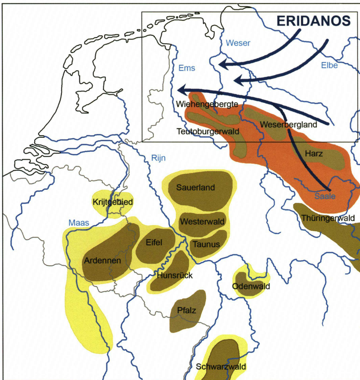
Tekstfig. 53. Herkomstgebieden van zwerfstenen. Zuidelijk van Rijn en Maas. Oostelijk van de Jonge Baltische Stroom. (H. Akkerman, 2010).
