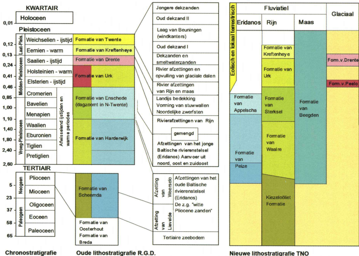
Tekstfig. 51. - Overzicht van de naast elkaar gezette lithostratigrafie van de R.G.D. en het TNO. In de tekst staan verwijzingen naar de nieuwe stratigrafie tussen haakjes. (H. Akkerman gewijzigd naar W.H. Zagwijn, 1975 en H. Weerts et al., 2008).
