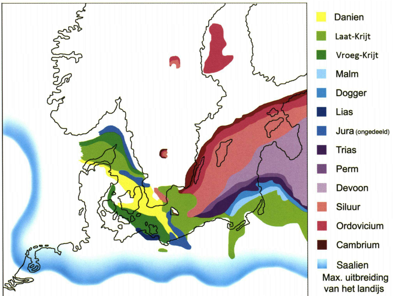
Tekstfig. 58. Herkomstgebieden van sedimentaire zwerfstenen uit Scandinavië en Noord-Duitsland. Glaciaal transport gedurende het Saalien. (H. Akkerman, gewijzigd naar W. Schulz, 2001).
