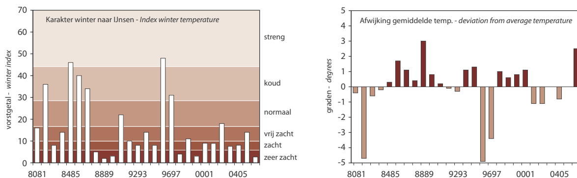
Figuur 4. Strengheid van de winter naar de terminologie van IJnsen (1991) en de gemiddelde temperatuur in december, uitgedrukt als afwijking van de normale temperatuur (gegevens KNMI, www.knmi.nl ). Index of winter temperatures according to the IJnsen-classification (ranging from 0 very mild to >50 severe winter) and average temperatures in December (counting period), expressed as deviation from normal values.
