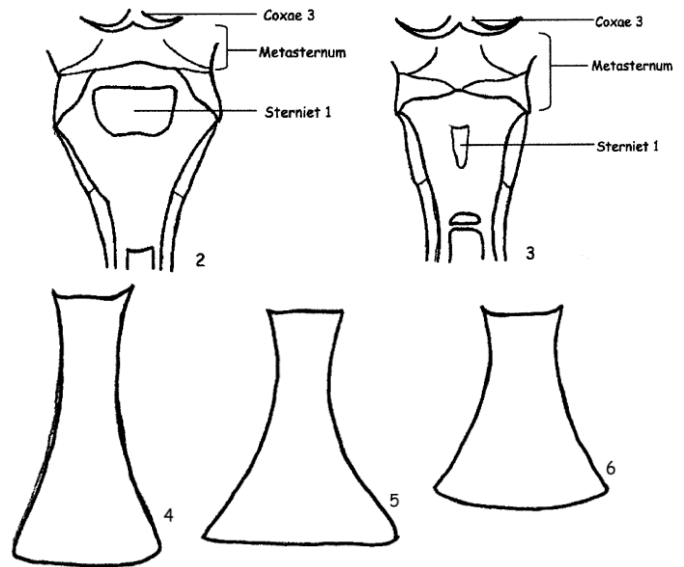
Figuur 2,3: Metasternum. 2: S. clunipes ; 3: S. sibirica .
