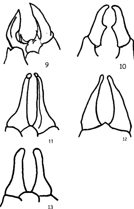
Figuur 9-13: genitaliën Sphegina . 9: S. sibirica ; 10: S. elegans ; 11: S. clunipes ; 12: S. clavata en 13: S. verecunda (naar Verlinden 1991).
